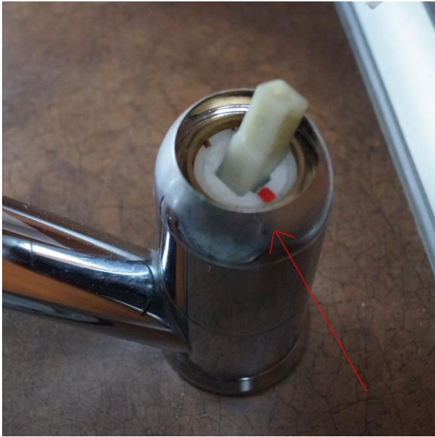
3) Pynteringen kan skrues af med håndkraft.
